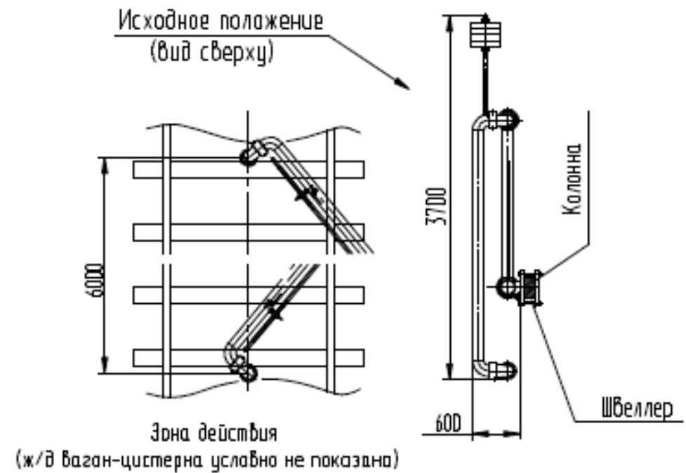
Монтажная схема
